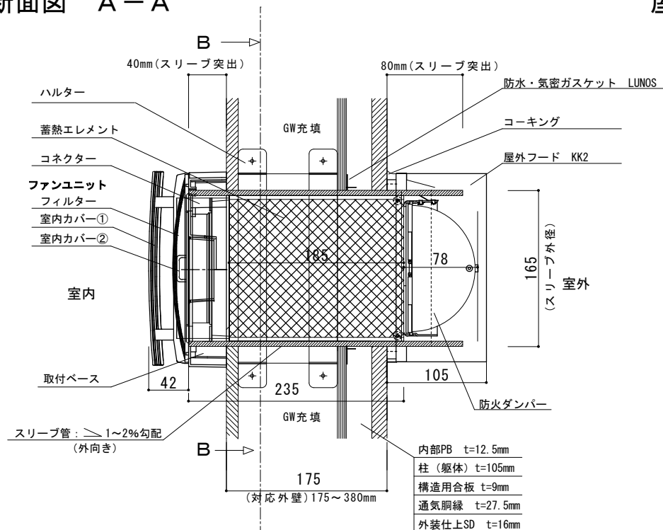
断面図 A-A
