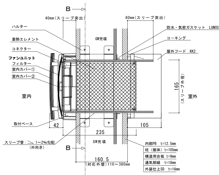
断面図 A-A
