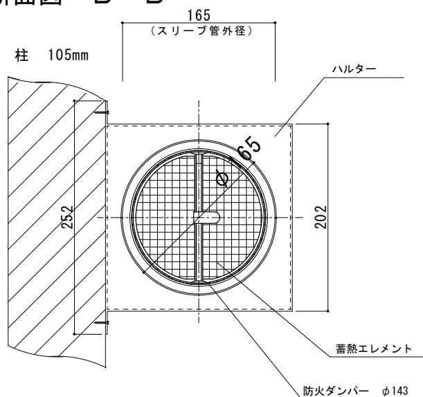
断面図 B-B
